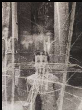
Espectro-grafía
